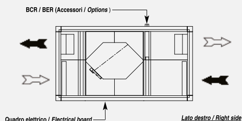
Mod. 40 Orientamento tipo 02 / Configuration type 02
