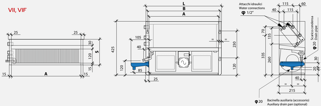
Dimensioni versioni verticali
