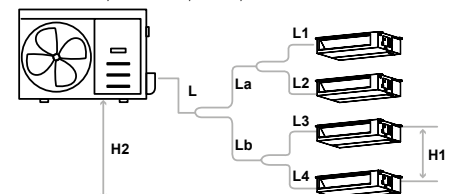
Sistema in parallelo quadruplo
